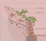
Opere stabilizzanti 14 - Gradonata
